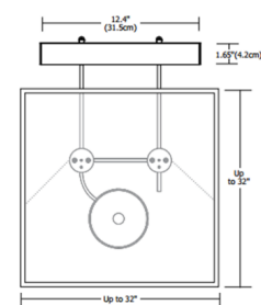
Cody 12" Canopy
