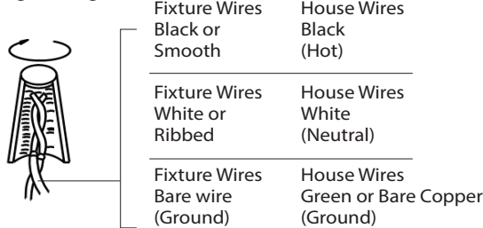
Fig. 2 Wiring
