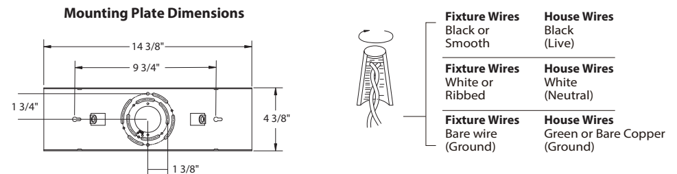
Fig. 2 Wiring
