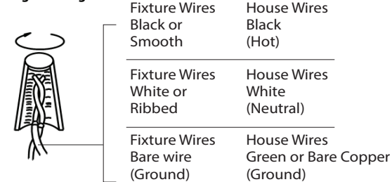
Fig. 2 Wiring
