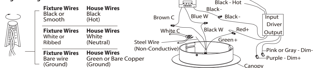
Fig. 2 Wiring
