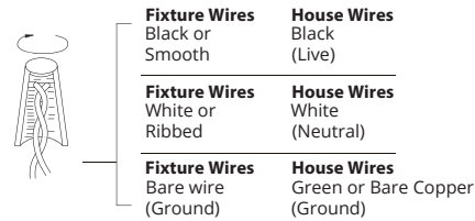
Fig. 2 Wiring
