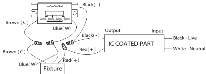
Fig. 3 Switch
