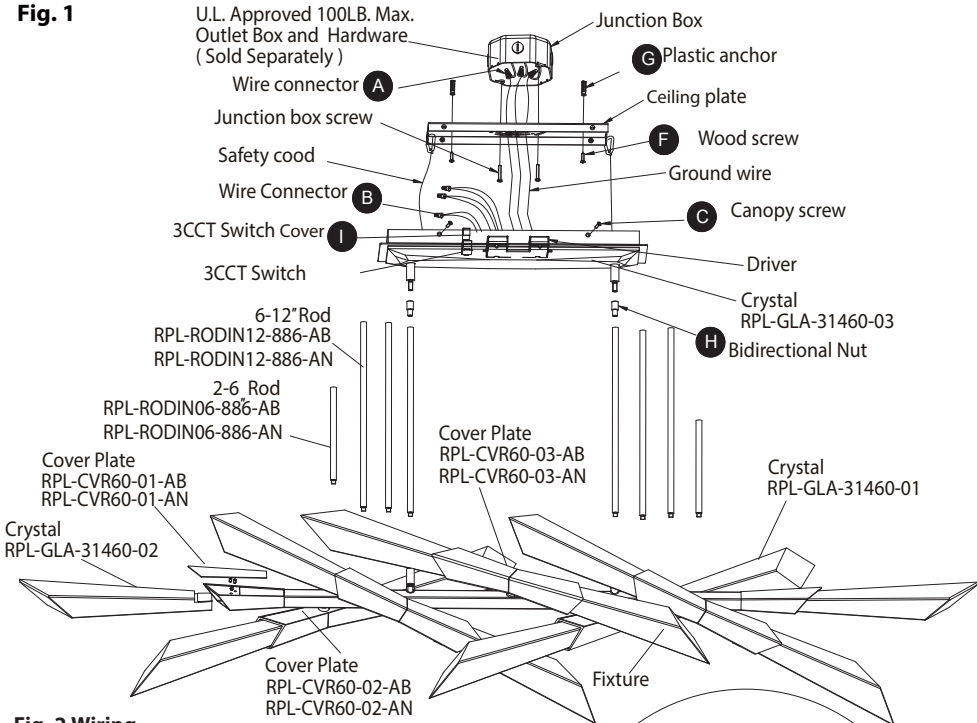
Fig. 2 Wiring
