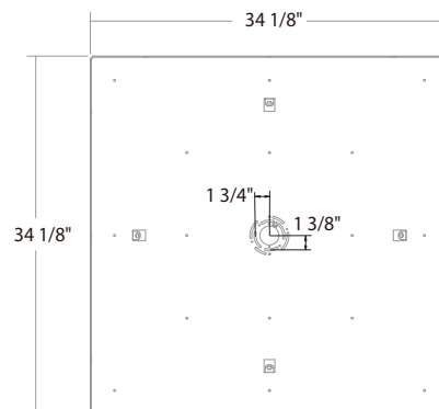
BPD-13241S
