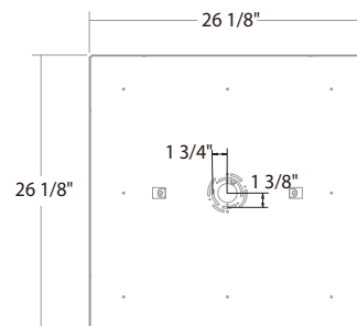
BPD-13225S
