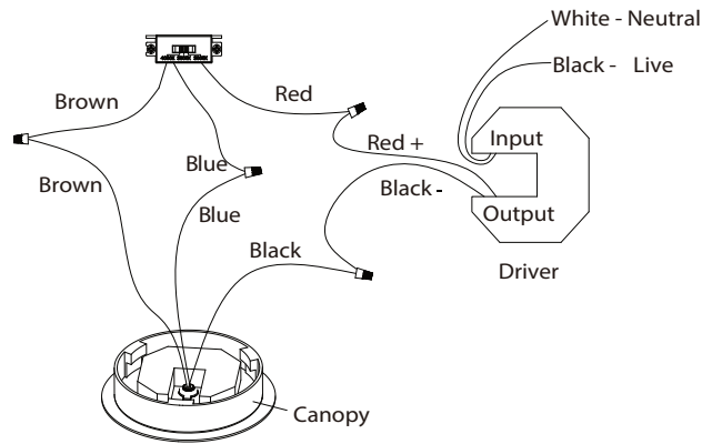
Fig. 4 Wiring
