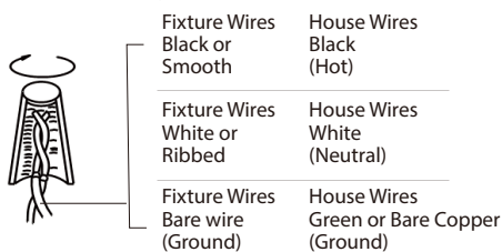
FIG. 3 Wiring
