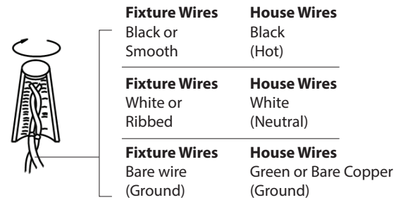
Fig. 2 Wiring
