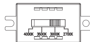
Fig. 3 Switch
