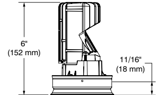
FLANGELESS TRIM
