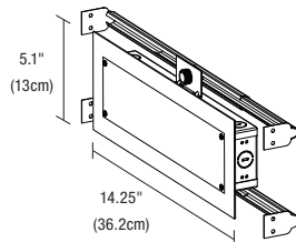
PSB-96W-010-24VDC-IW
