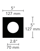
FLANGELESS
