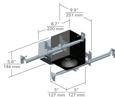
IC AIRTIGHT / NON-IC AIRTIGHT (MAX CEILING THICKNESS: 2")
