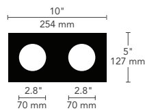
FLANGELESS
