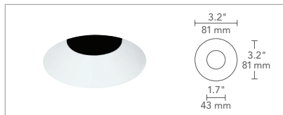
FLANGELESS BEVEL
