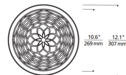
TORUS FLANGELESS 12"
