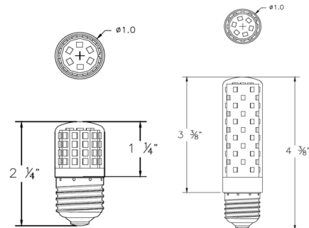
E26 3.0W Amber
