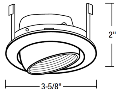
Trim OD: 3-5/8"
