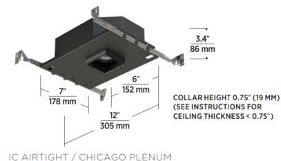
IC AIRTIGHT / CHICAGO PLENUM
