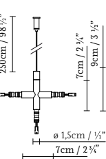
KUPETZ X S
